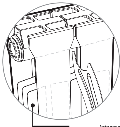
Intermediate fins
